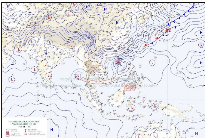
แผนที่อากาศ วันที่ ๑๒ ก.ย. ๒๕๖๙ เวลา ๐๑.๐๐ น.
