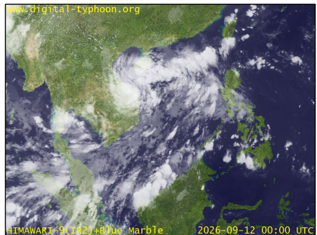
ภาพถ่ายดาวเทียม วันที่ ๑๒ ก.ย. ๒๕๖๙ เวลา ๐๗.๐๐ น.
